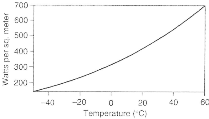
الشكل ١-٢ القوة الكلية التى يشعها جسم أسود بوصفها دالة لدرجة الحرارة وات/م ٢ .
